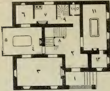
( روشن قات پلانی )
